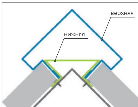
Наружный сборный угол 3D (Рис. 1)
