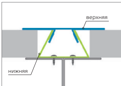
Соединение панелей (Рис. 3)
